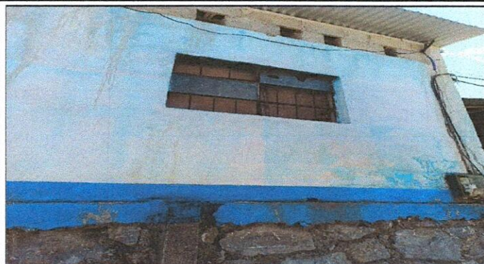
Foto 13: Remodelación en estructura de metal en ventana de la cocina
