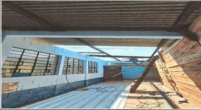
Foto 1: Cambio de lámina troquelada Calibre 26
